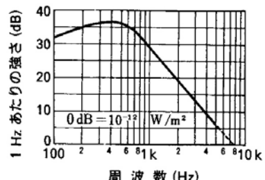
図 話声の長時間平均スペクトル (出典: 参考文献 [2], p.21)
