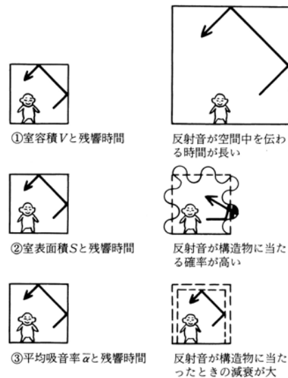
図 残響予測式の定性的理解 (出典: 参考文献 [1], p. 116)
