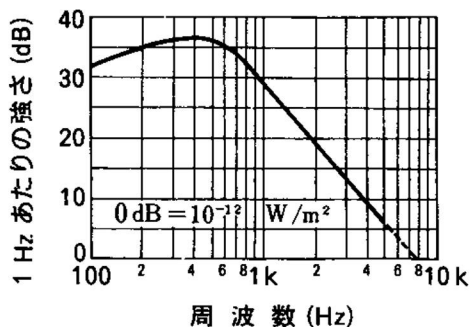
図 話声の長時間平均スペクトル
